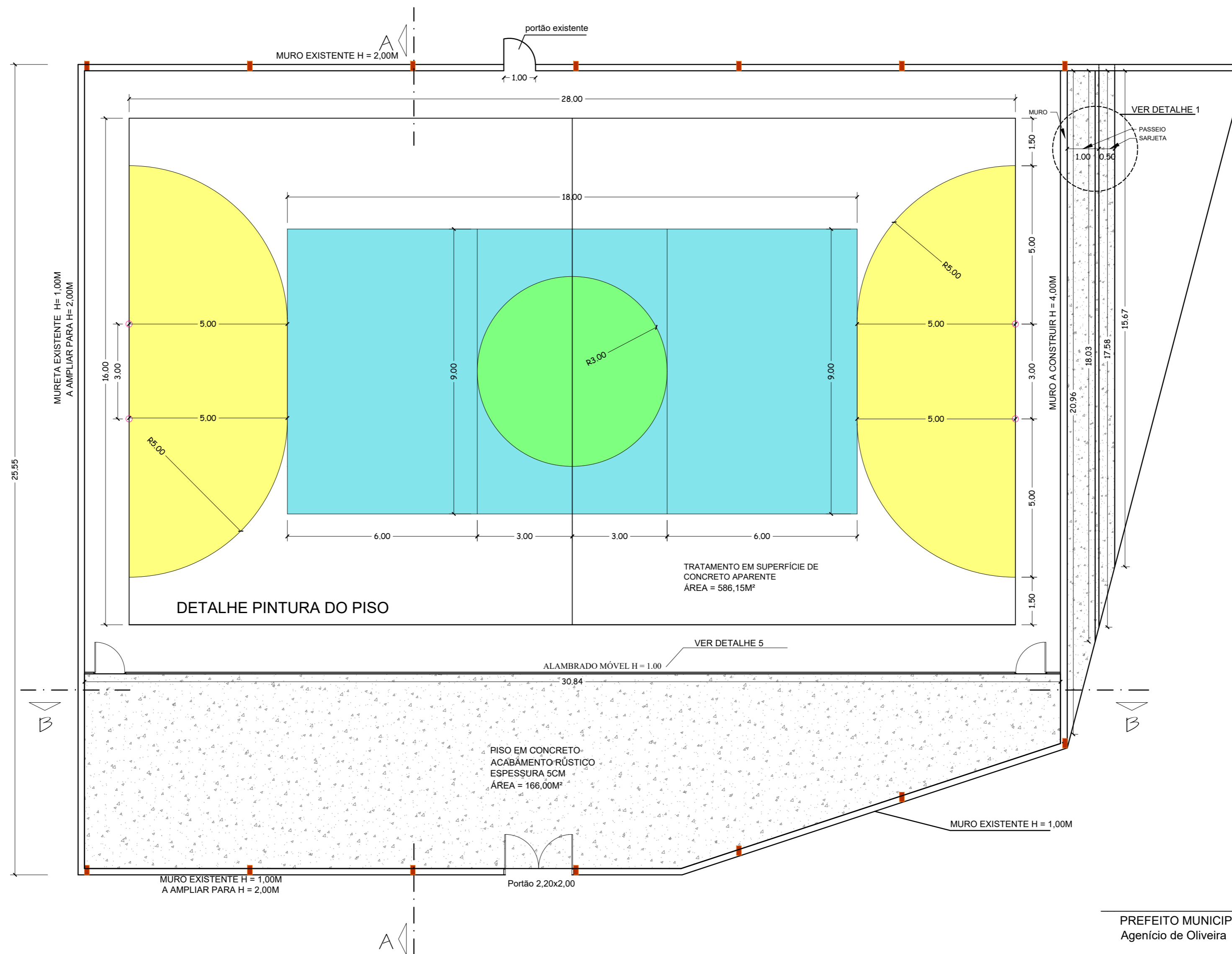
PLANTA BAIXA QUADRA POLIESPORTIVA ESCALA 1:100
