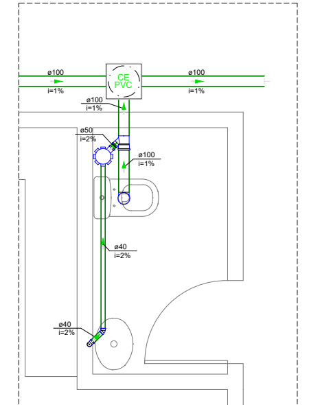
DETALHE SAN-3 1:25
