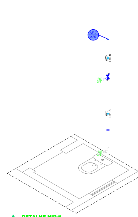
DETALHE HID-6 1:25
