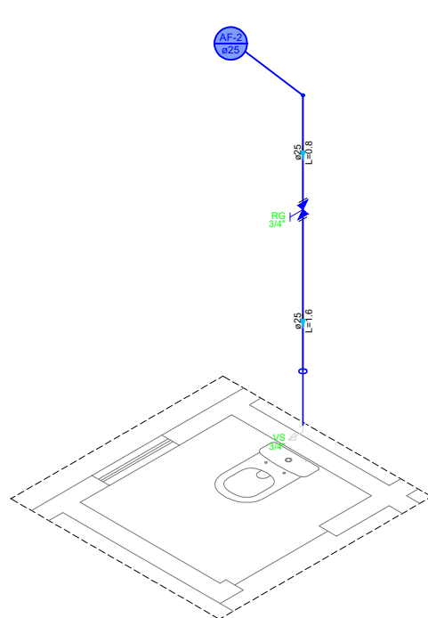
DETALHE HID-2 1:25
