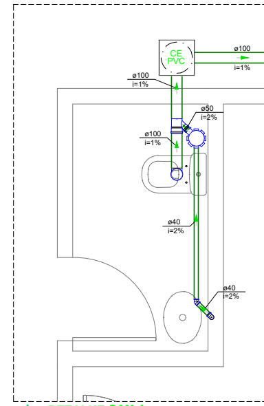
DETALHE SAN-1 1:25
