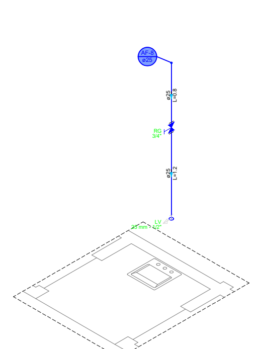
DETALHE HID-7 1:25
