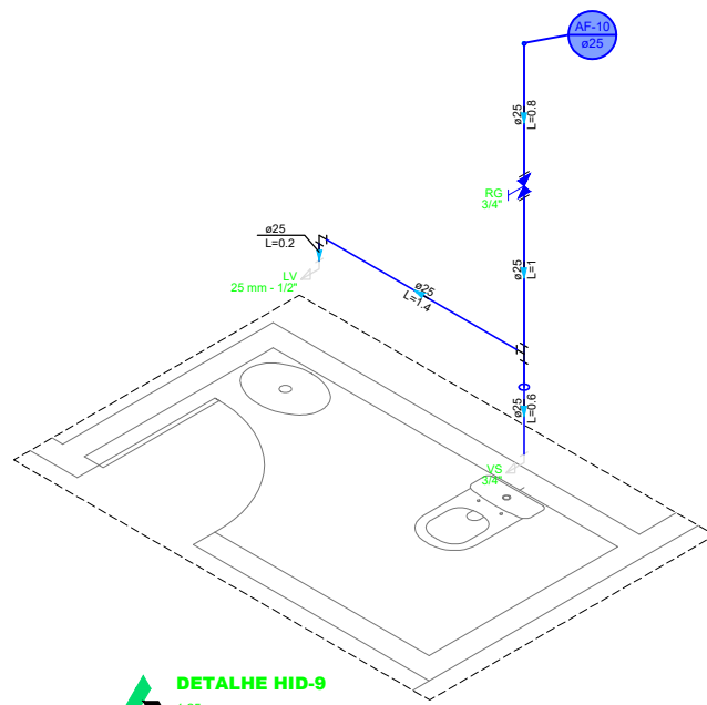
DETALHE HID-9 1:25
