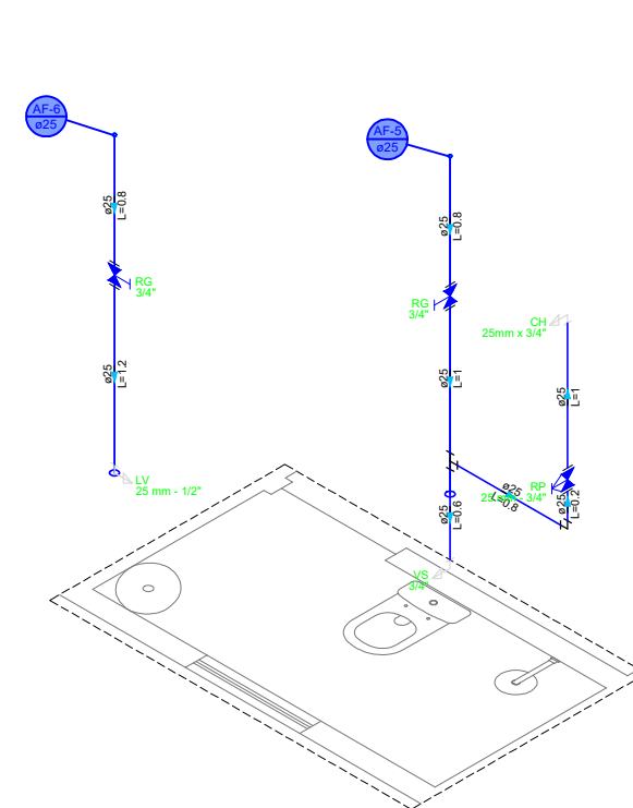
DETALHE HID-5 1:25
