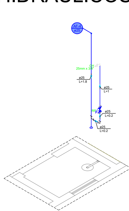
DETALHE HID-4 1:25
