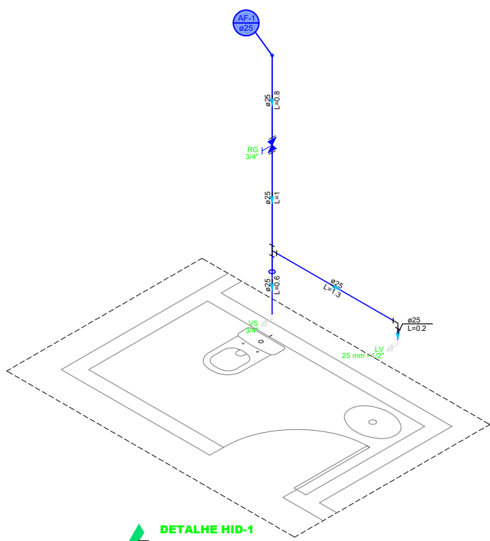
DETALHE HID-1 1:25
