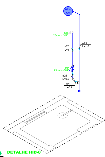
DETALHE HID-8 1:25
