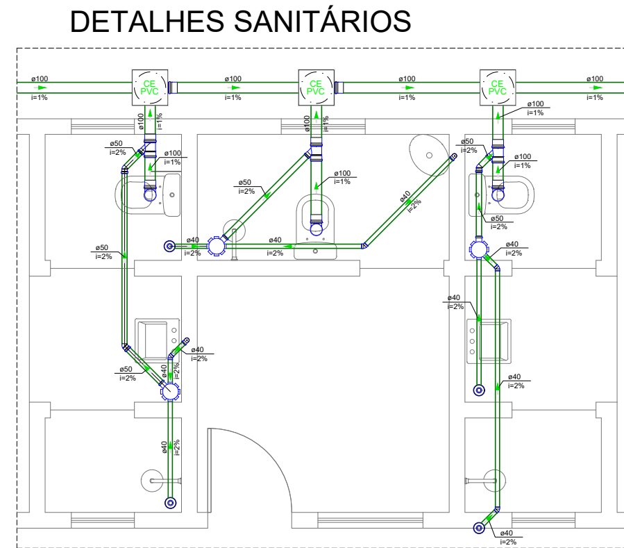
DETALHE SAN-2 1:25
