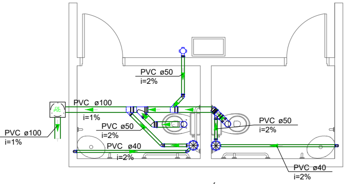
1 PLANTA DO PAVIMENTO TÉRREO INSTALAÇÕES SANITÁRIAS ESC - 1:25
