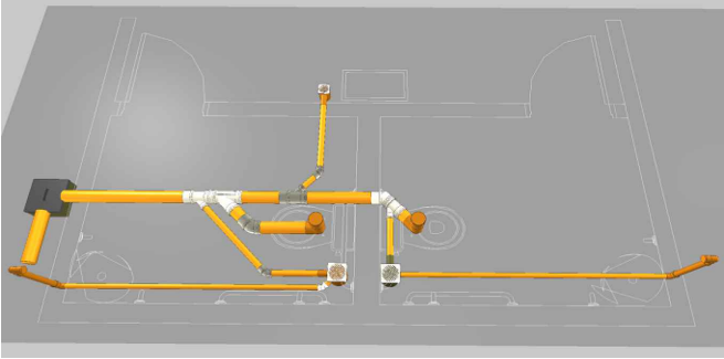
2 PLANTA DO PAVIMENTO TÉRREO INSTALAÇÕES SANITÁRIAS DETALHE 3D
