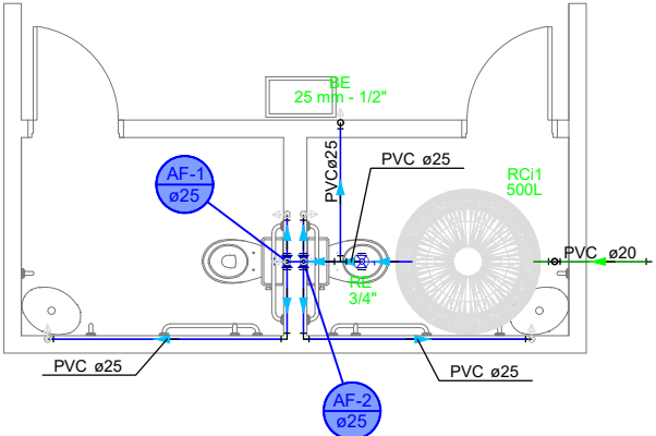
1 PLANTA DO PAVIMENTO TÉRREO INSTALAÇÕES HIDRÁULICAS ESC - 1:25
