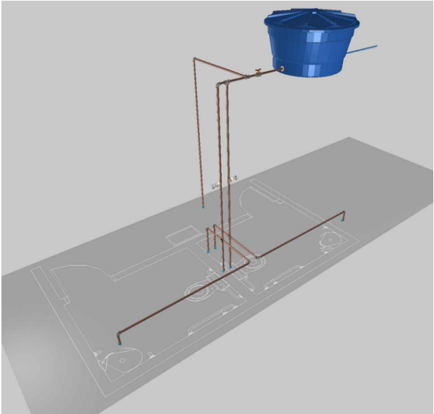
2 PLANTA DO PAVIMENTO TÉRREO INSTALAÇÕES HIDRÁULICAS DETALHE 3D
